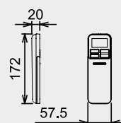
Telecomando infrarossi
