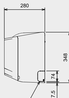
Sistema knock out
