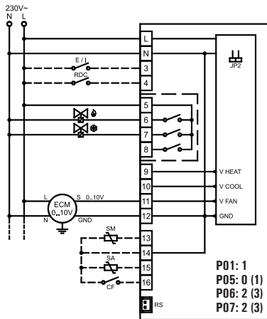
Fig. 8: Schema di collegamento per pilotaggio di due attuatori on/off a 230V ~ per impianto a 4 tubi e pilotaggio proporzionale del ventilatore. Wiring diagram for 2 on/off 230V ~ actuators in 4 pipes system and proportional fan drive.
